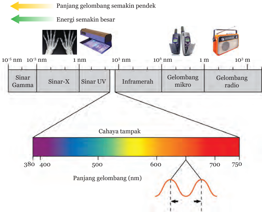
Gambar 11.8 Spektrum Elektromagnetik
