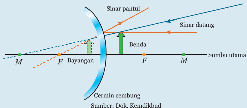
Gambar 11.21 Gambar Diagram Sinar pada Cermin Cembung
